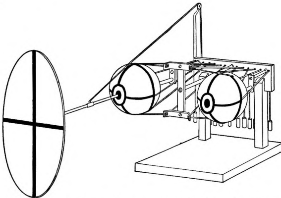
FIG. 23.—Ophthalmotrope (Zimmermann, Mk. 64). See Helmholtz, Phys. Optik , 1896, 667.
