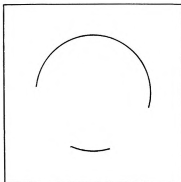
FIG. 47. — Müller-Lyer.
