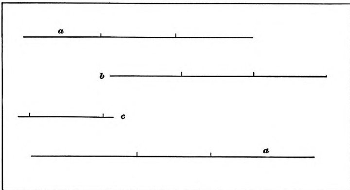
FIG. 43. — Wundt.
