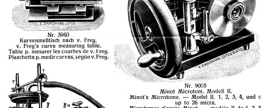
Nr. 2900 Sphigmyograph nach Marej. Marej's Sphigmyograph. — Sphigmyographie de Marej. Esfigmógrafo según Marej. Nr. 9010 Mikrotom Minot. Modell III. Same thicknesses of slices as model II, and additional 6, 13, 20, 26, 33, and 40 micra. épaisseurs égales des coupes comme modèle II et autres de 6, 13, 20, 26, 33 et 40 microns. Espesores de corte iguales a los del modelo II y otros de 6, 13, 20, 26, 33 y 40 microns.
