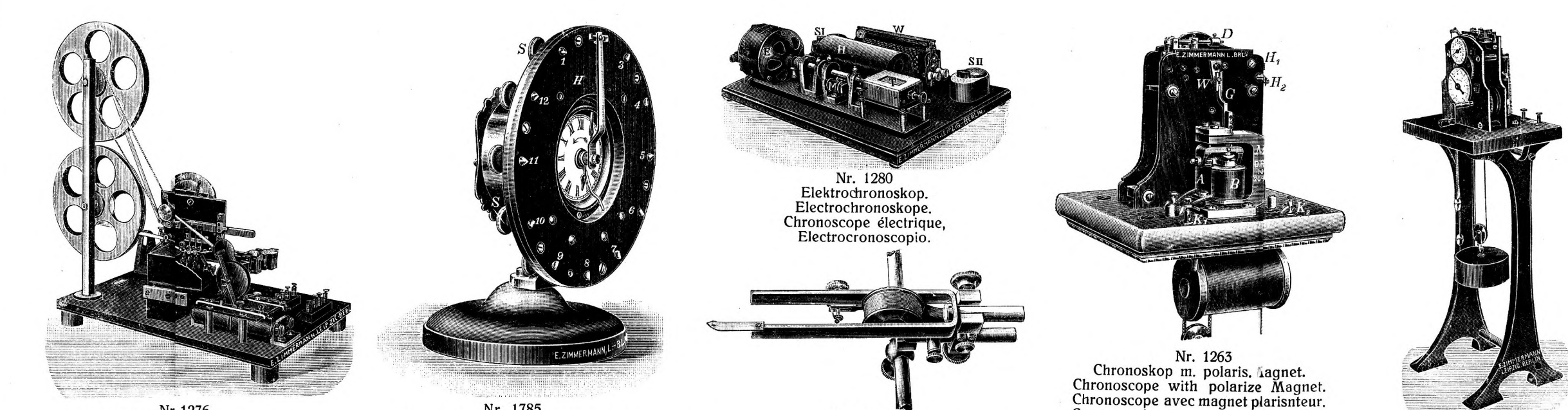
Nr. 1263 Chronoskop m. polaris. magnet. Chronoscope with polarizer Magnet. Chronoscope avec magnet polarisateur. Cronoscopio cou magneto polarizador. Nr. 1261 Chronoskop nach Hipp. Hipp's chronoscope. Chronoscopo de Hipp. Nr. 1290 Elektrochronoskop. Electrochronoscope. Electrocronoscopio. Nr. 1785 Kontaktuhr für größere Intervalle. Contact clock for larger intervals. Pendule p. grands intervalles. Reloj de contacto p grandes intervalles. Nr. 1703 Elektromagn. Stimmgabel f. dir. Zeitschreibung. Electromagn. tuning fork f. dir. time-recording. Diapason p. l'enregist. direct du temps. Diapason electromagn. p. inscrip. directa d. temps. Nr. 1216 Zählender Chronograph nach Lewin. Lewin's counting Chronograph. Chronographe de Lewin. Cronografo contador Lewin.
